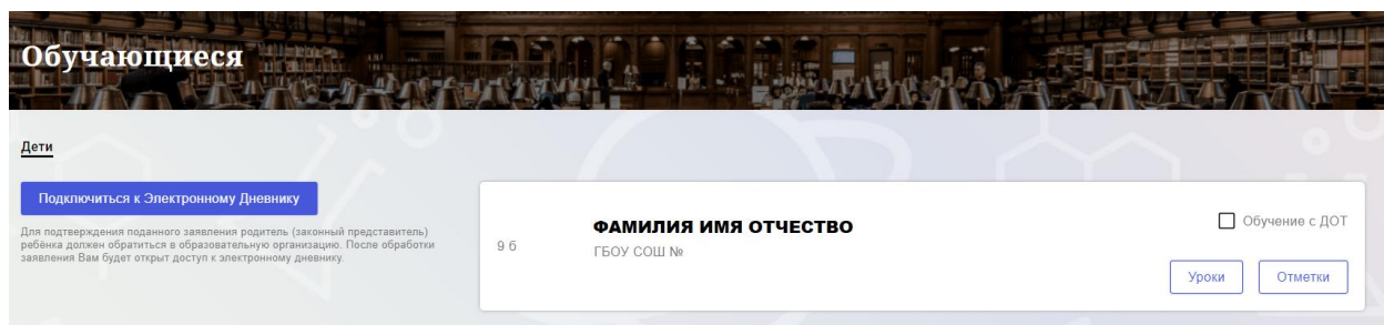
Рисунок 8 – Страница «Обучающиеся»
